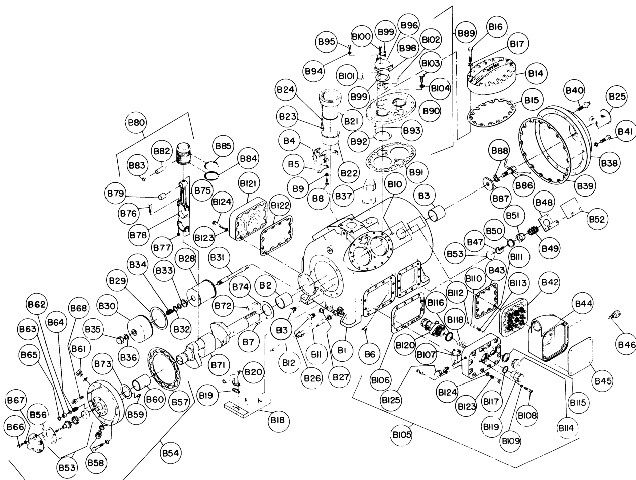
6G45 SHOWN
