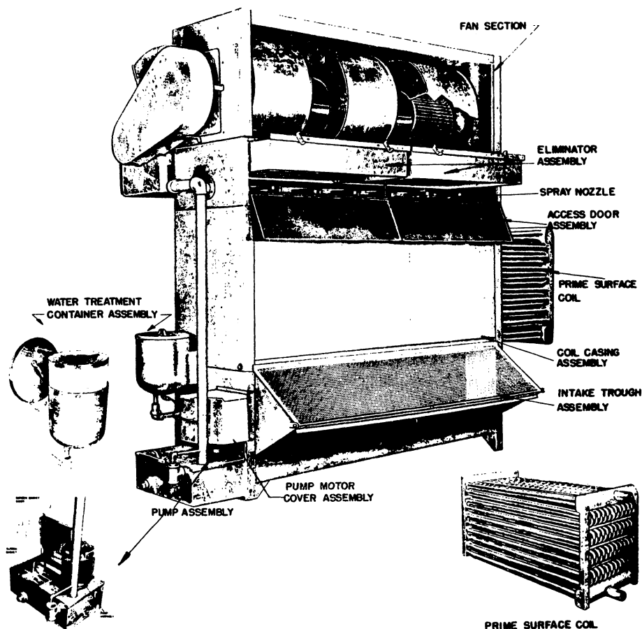
9E EVAPORATIVE CONDENSER
