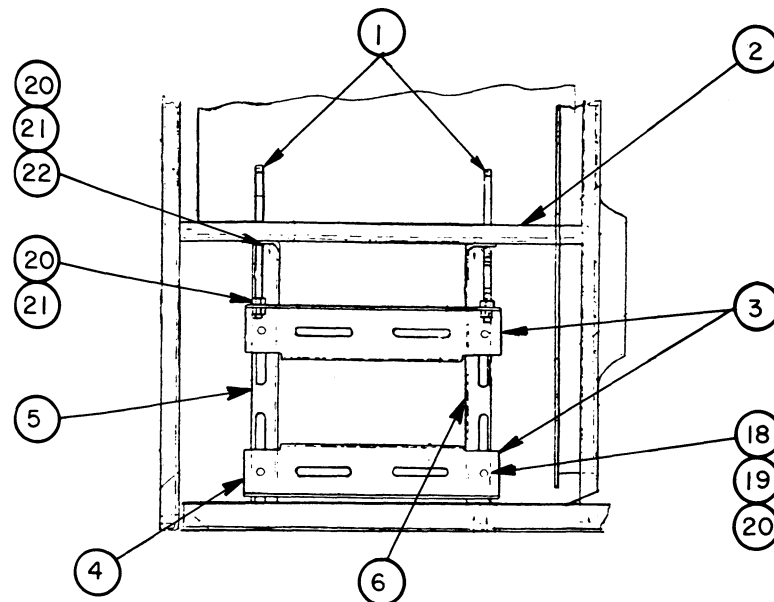
MOTOR BASE ASSEMBLY (T.H.F. & U.B.F.) L.H. UNIT
