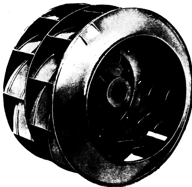
AIRFOIL FAN
