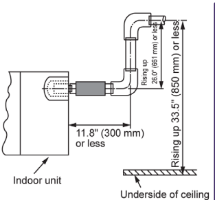
3x3 Cassette
